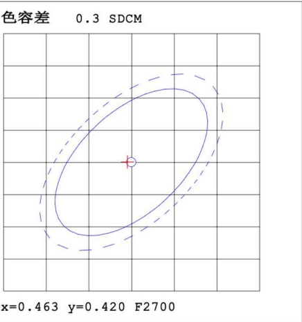
CIE1931色品图
