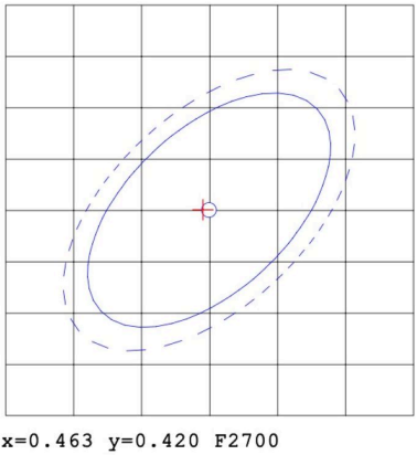
CIE1931色品图
