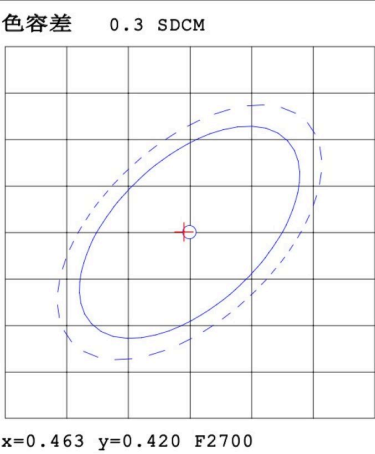
CIE1931色品图
